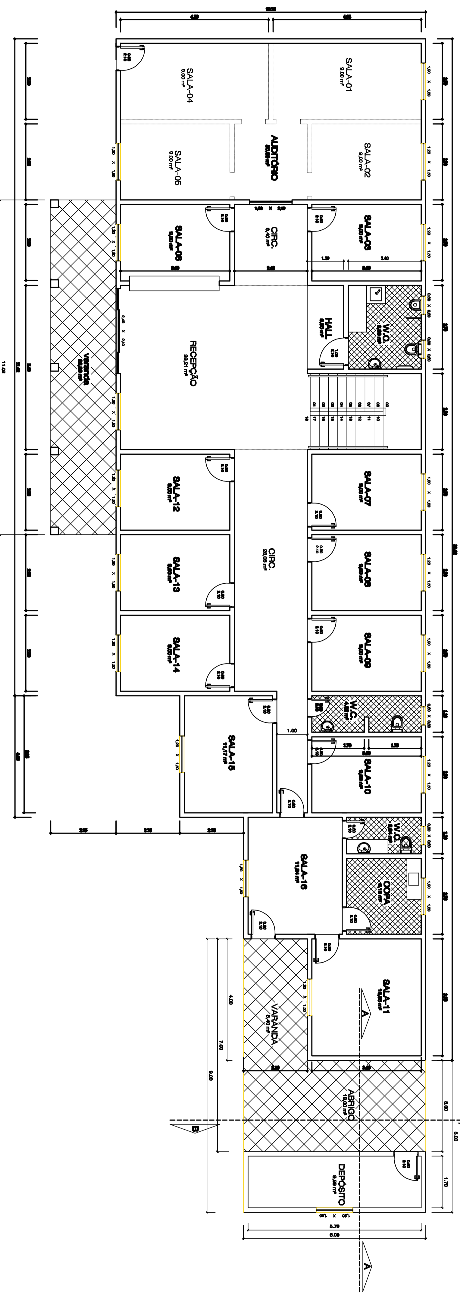
PLANTA BAVA - 1º PAVT ESCALA ..... 1/80
